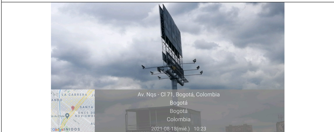
Foto 2. Vista del panel, del mástil y de la estructura de la valla, en buenas condiciones y estable.
